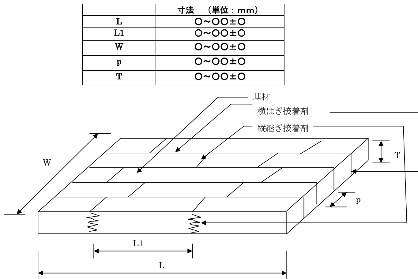
断面図例
